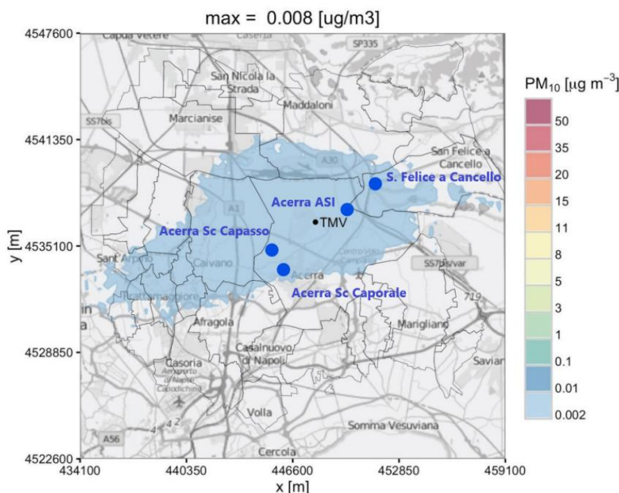
FIGURA 1: 90.4° PERCENTILE DELLE MEDIE GIORNALIERE DI PM10 EMESSO DAL TERMOVALORIZZATORE DI ACERRA (TMV). IN BLU SONO INDICATE LE QUATTRO STAZIONI DI MONITORAGGIO DELLA QUALITÀ DELL'ARIA GESTITE DA ARPAC.
