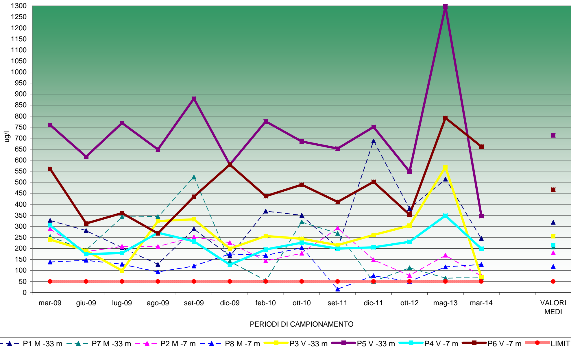
GRAFICO N. 13 INCENERITORE CON RECUPERO DI ENERGIA DI ACERRA (NA) ANDAMENTO DELLA CONCENTRAZIONE DI MANGANESE NEL PERIODO MARZO 2009-MARZO 2014 NELLE FALDE SUPERFICIALI (-7 m) E PROFONDE (-33 m) A MONTE (M) E VALLE (V)
