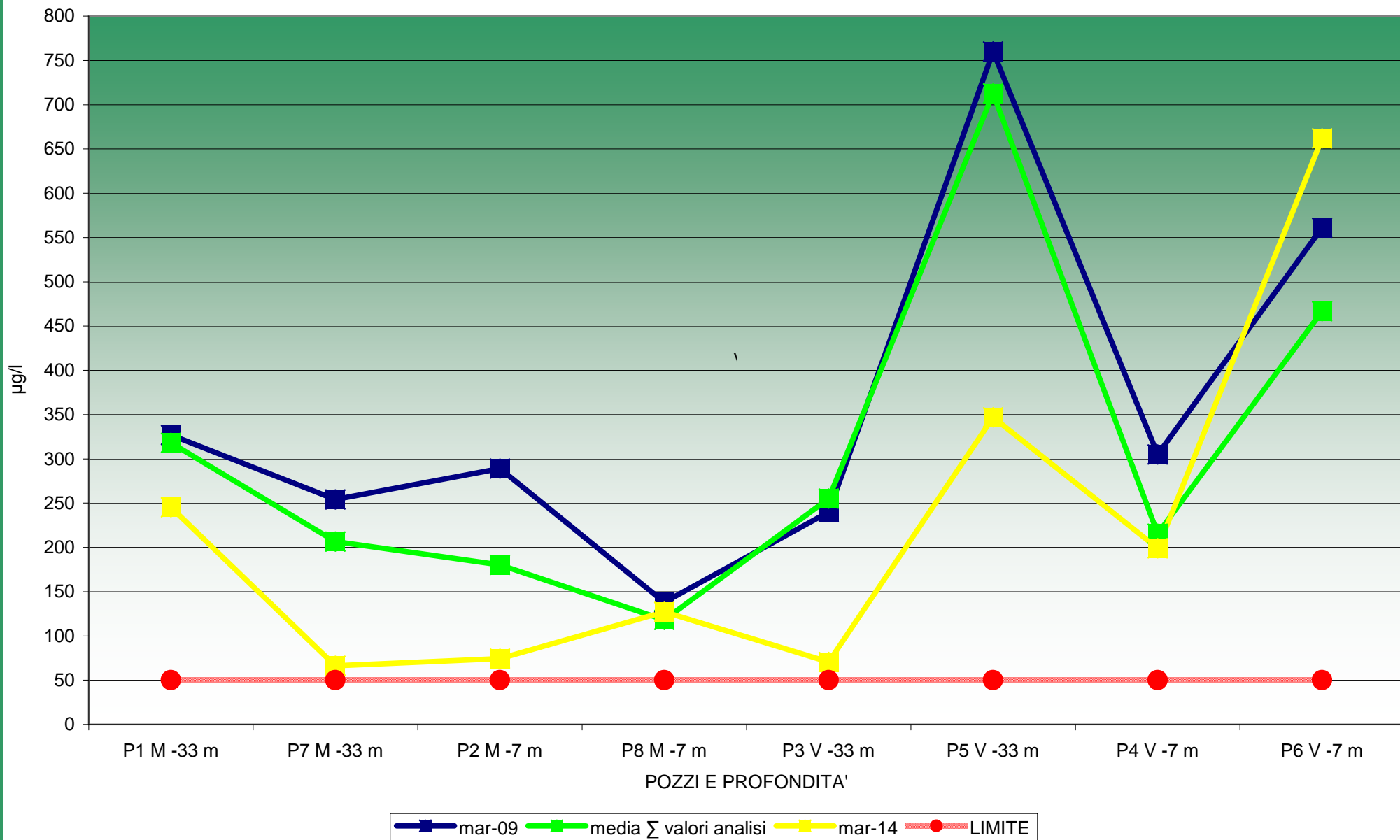
GRAFICO N. 14 INCENERITORE CON RECUPERO DI ENERGIA DI ACERRA (NA) CONFRONTO DI MANGANESE IN FALDE SUPERFICIALI (-7 m) - PROFONDE (-33 m) - MONTE (M) - VALLE (V) TRA BIANCO AMBIENTALE (MARZO 2009) ULTIMA VERIFICA (MARZO 2014) E MEDIA \Sigma VALORI ANALISI
