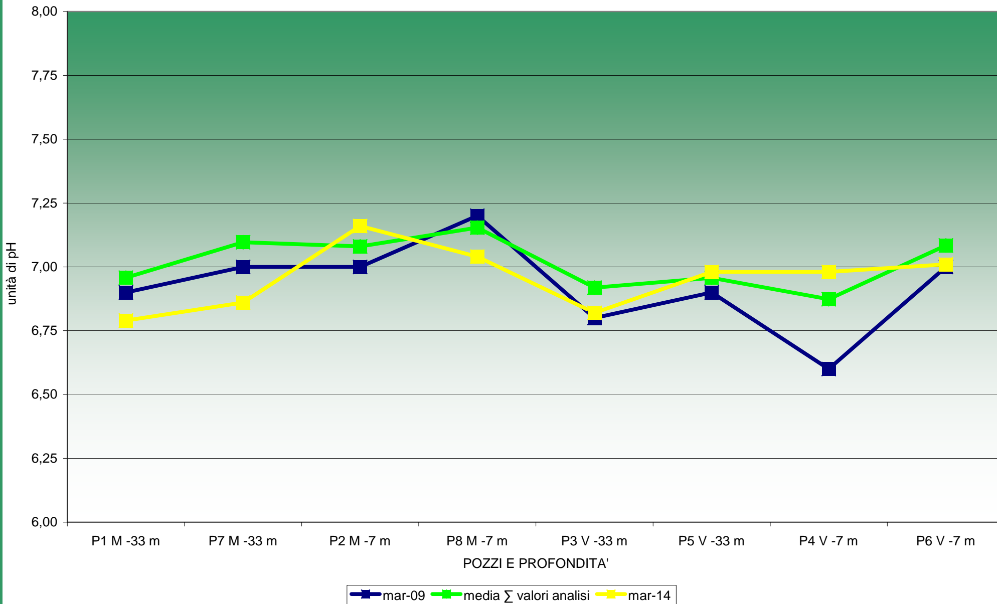
GRAFICO N. 18 INCENERITORE CON RECUPERO DI ENERGIA DI ACERRA (NA) CONFRONTO DEL pH IN FALDE SUPERFICIALI (-7 m) - PROFONDE (-33 m) - MONTE (M) - VALLE (V) TRA BIANCO AMBIENTALE (MARZO 2009) ULTIMA VERIFICA (MARZO 2014) E MEDIA \Sigma VALORI ANALISI
