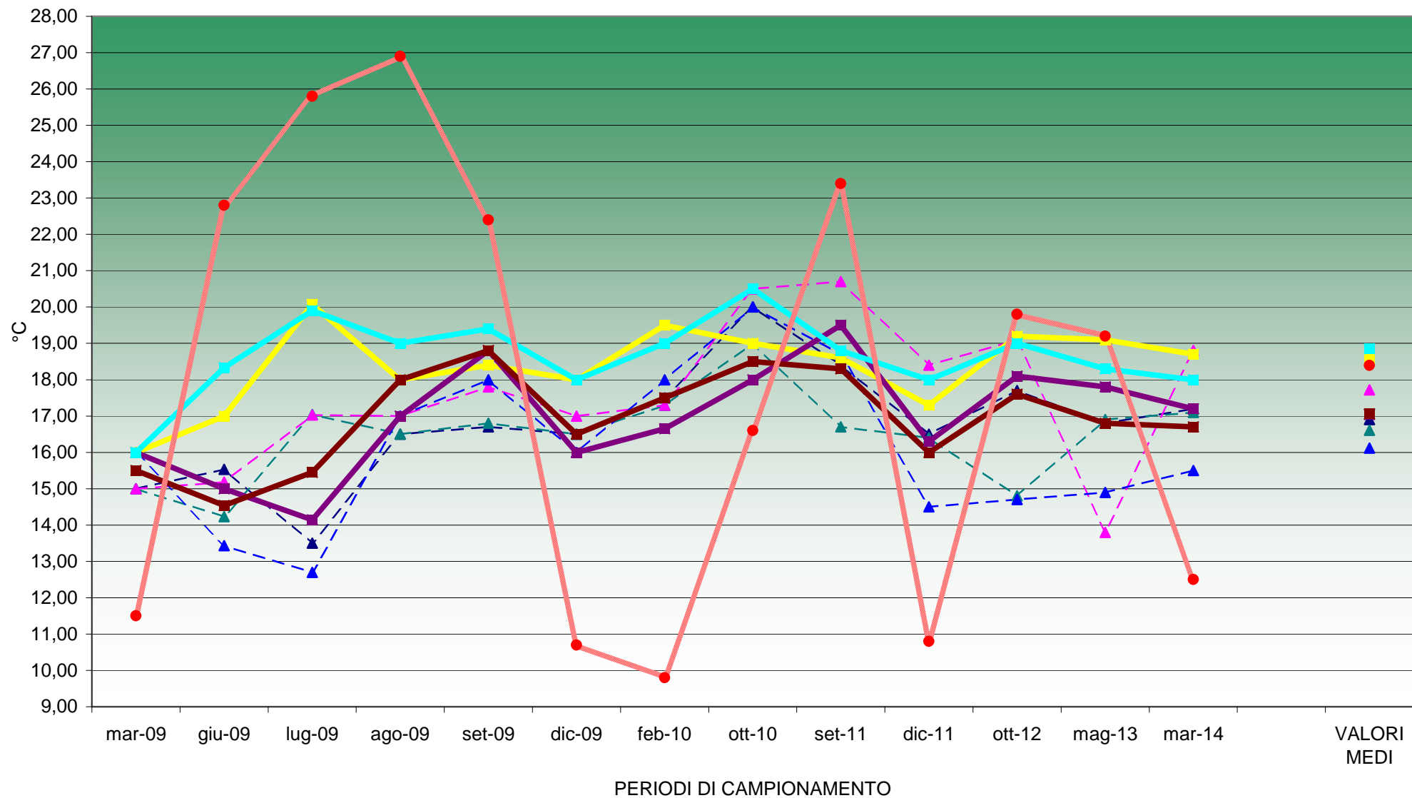
GRAFICO N. 19 INCENERITORE CON RECUPERO DI ENERGIA DI ACERRA (NA) ANDAMENTO DELLA TEMPERATURA NEL PERIODO MARZO 2009-MARZO 2014 NELLE FALDE SUPERFICIALI (-7 m) E PROFONDE (-33 m) A MONTE (M) E VALLE (V)
