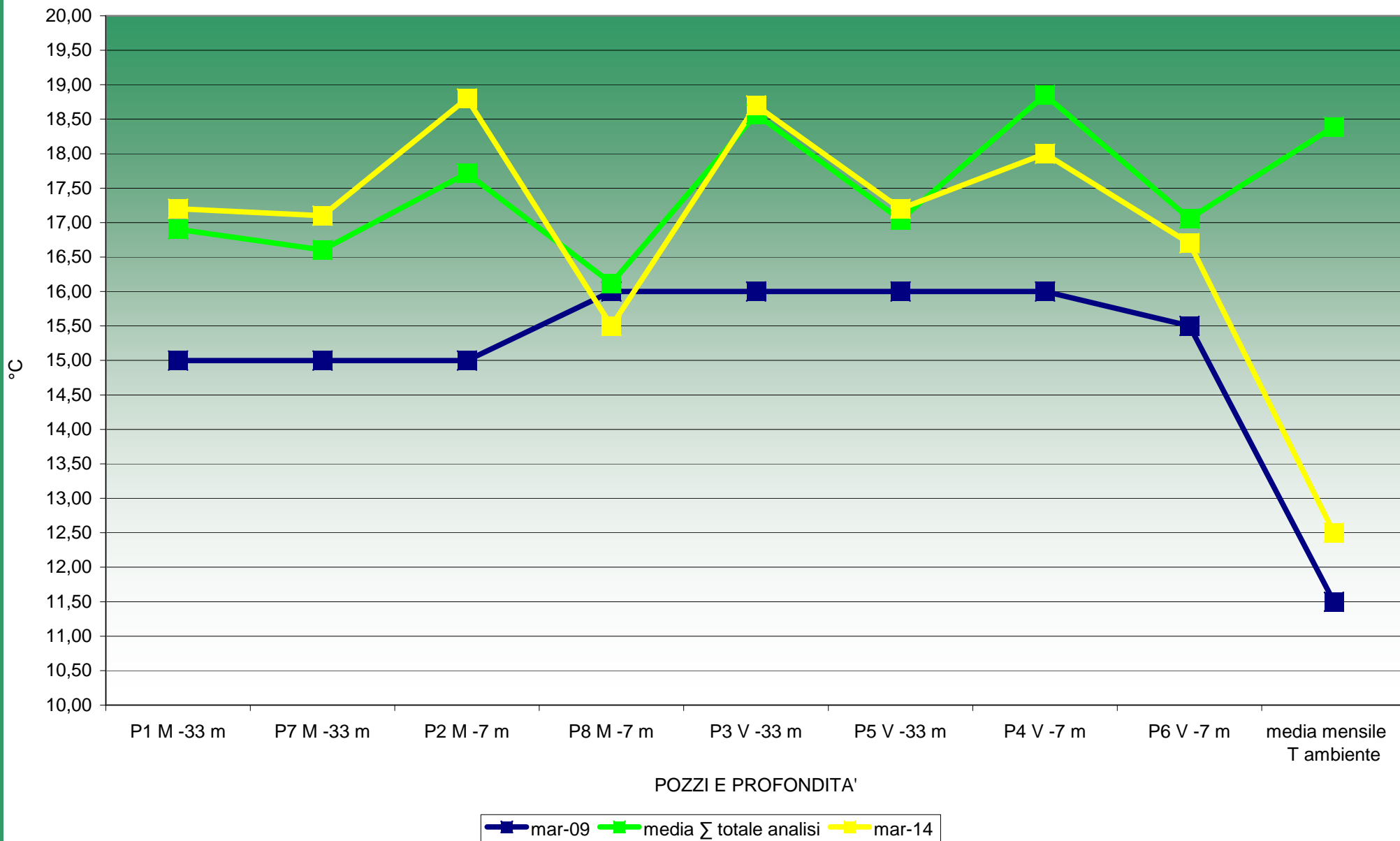
GRAFICO N. 20 INCENERITORE CON RECUPERO DI ENERGIA DI ACERRA (NA) CONFRONTO TEMPERATURA IN FALDE SUPERFICIALI (-7 m) - PROFONDE (-33 m) - MONTE (M) - VALLE (V) TRA BIANCO AMBIENTALE (MARZO 2009) ULTIMA VERIFICA (MARZO 2014) E MEDIA \Sigma VALORI ANALISI
